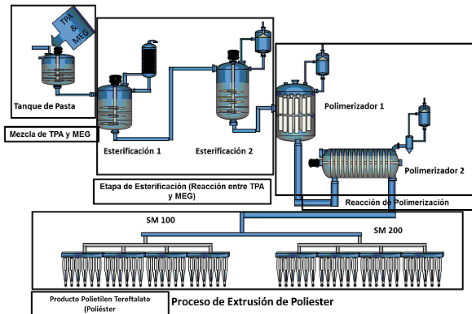
Proceso de reacción del poliéster esquematizado por reactores
