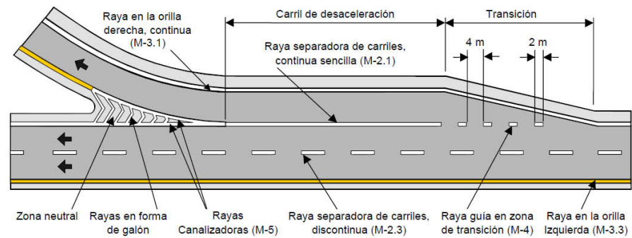
FIGURA 6.- Diversos tipos de rayas y marcas en el pavimento en aproximaciones de intersección
