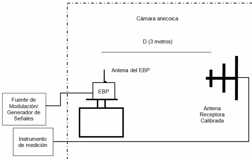
Figura 2. Configuración para medición de emisiones radiadas.
